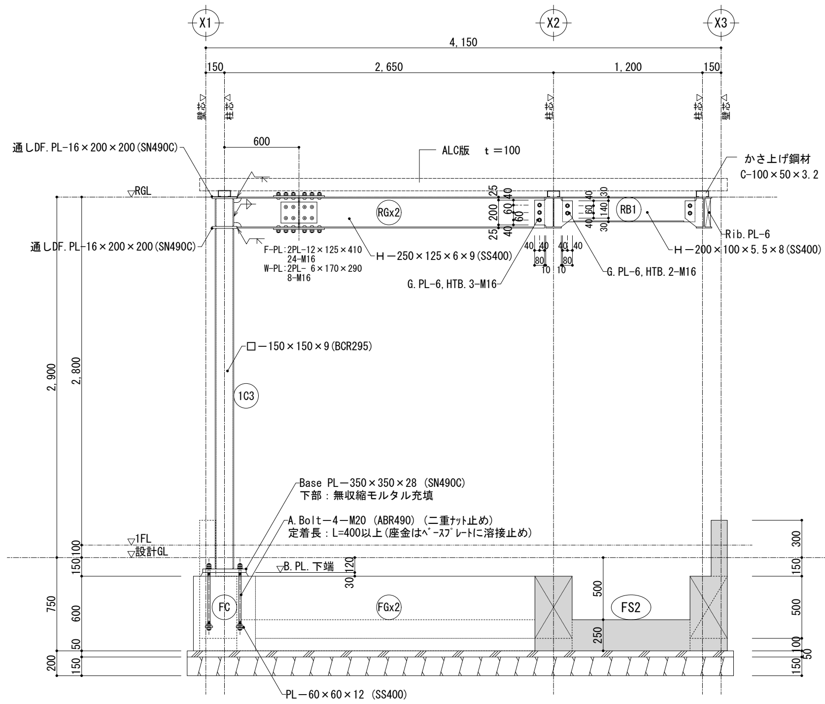
Y3通り架構詳細図 S=1:30
